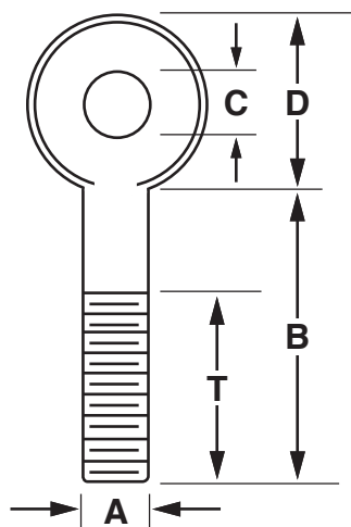
Rod End
